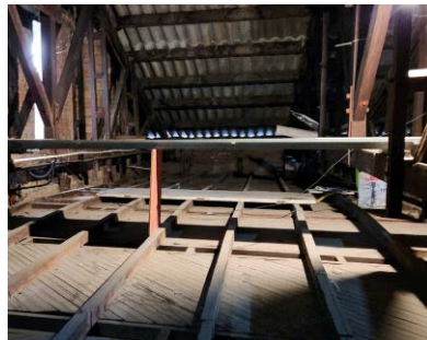
Troca das estruturas em madeira e alvenaria que dão suporte ao telhado.
